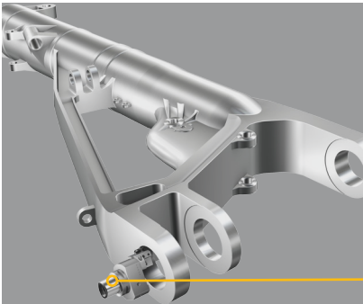
İniş takımı
