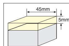
Material: SCM415 V=300m/min. f=0.3mm/tooth S=3800min -1 F=4560mm/min.
